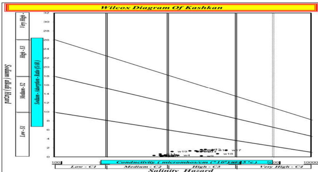
شکل ۳: طبقه‌بندی ویلکاکس برای رودخانه‌ی کشکان-ایستگاه پلدختر از سال ۷۵-۹۵
